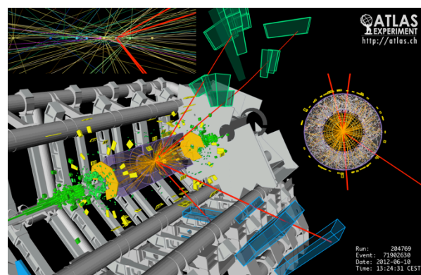
Abbildung 2. Kandidat für einen Higgs-Zerfall in vier Muonen, 2012 von ATLAS aufgezeichnet.
